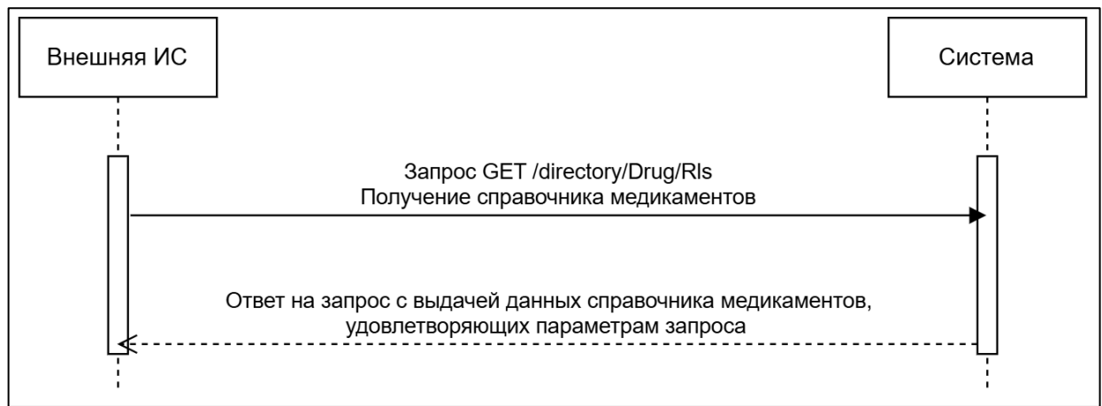
Рисунок 5 – Схема взаимодействия в части передачи справочника медикаментов
