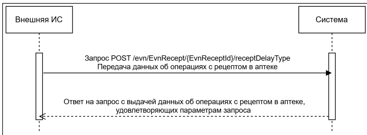
Рисунок 4 – Схема взаимодействия в части получения данных об операциях с рецептом в аптеке
