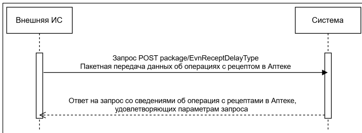
Рисунок 3 – Схема взаимодействия в части пакетного получения данных об операциях с рецептом в аптеке
