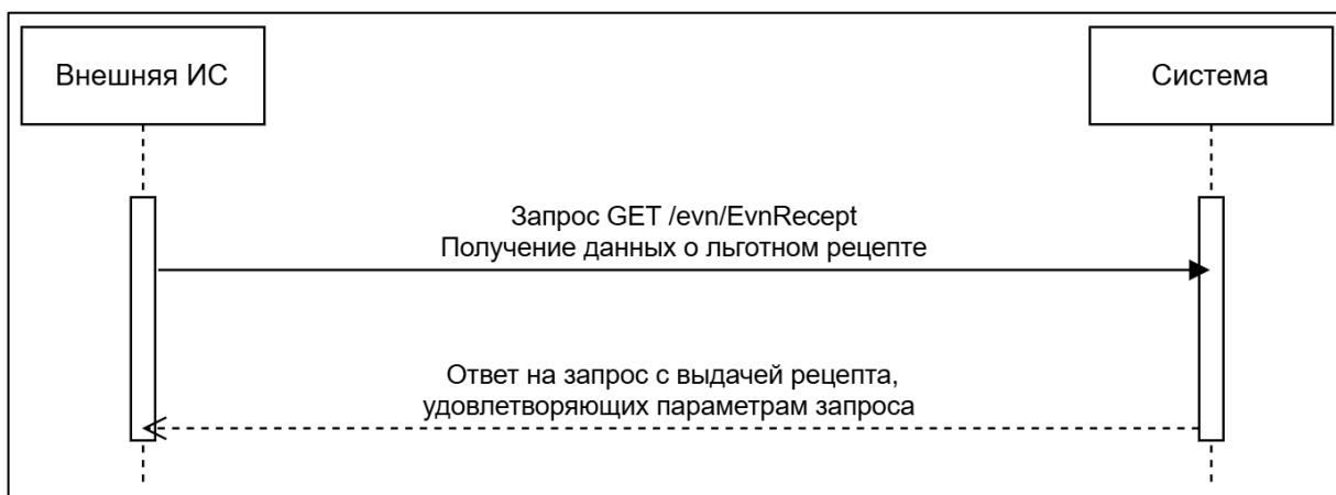
Рисунок 2 – Схема взаимодействия в части передачи данных о льготном рецепте
