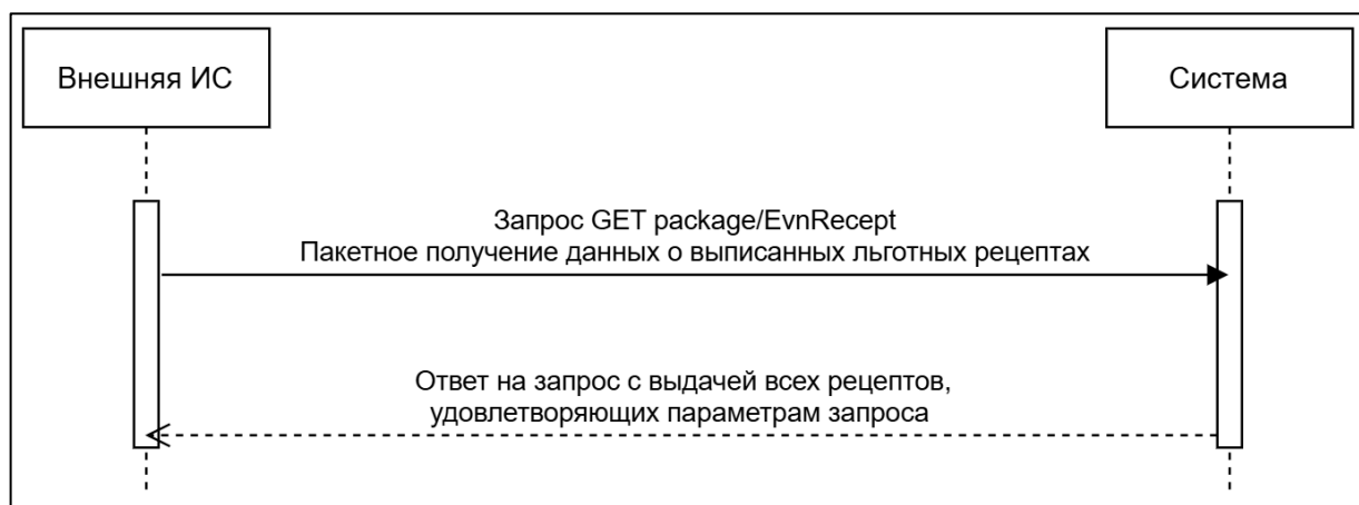
Рисунок 1 – Схема взаимодействия в части пакетной передачи данных о выписанных льготных рецептах
